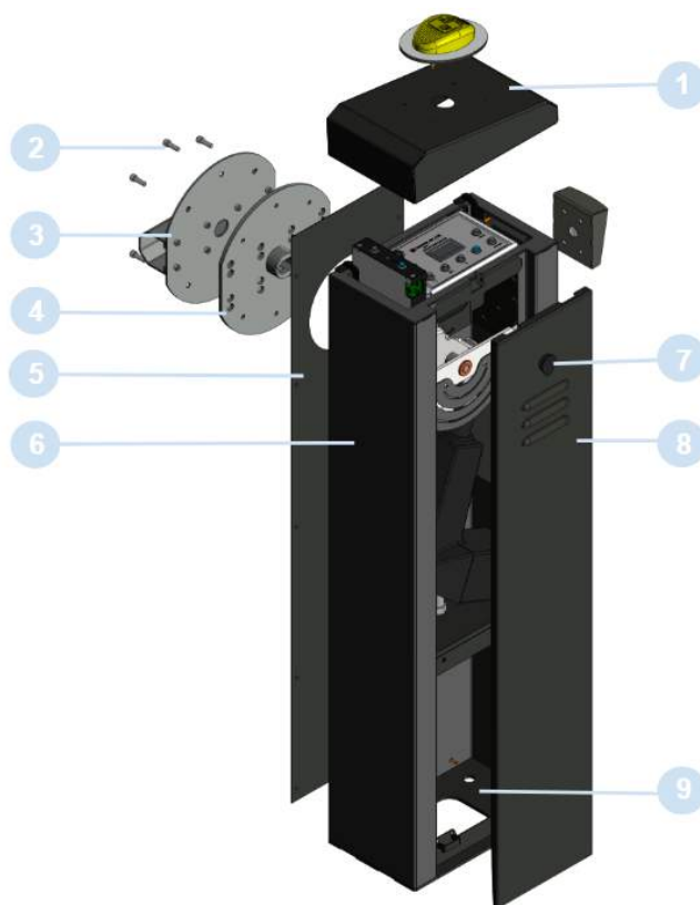
Рисунок 4. Внешний вид и состав корпуса шлагбаума
