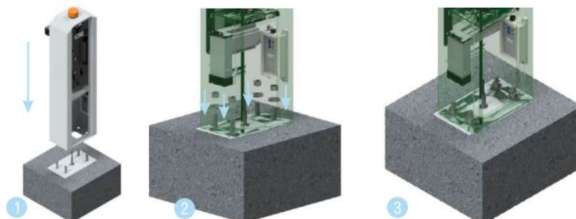
Рисунок 22. Установка тумбы шлагбаума
