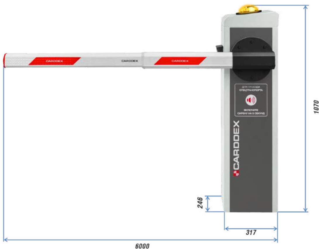
Рисунок 2. Габаритные размеры шлагбаума
