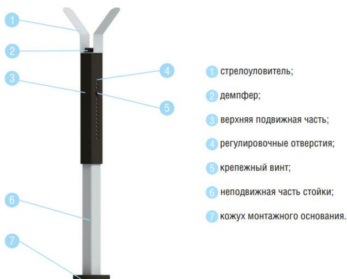
Рисунок 24. Опора стрелы
