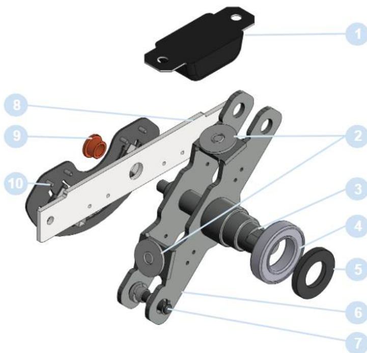
Рисунок 5. Узел крепления и управления стрелой
