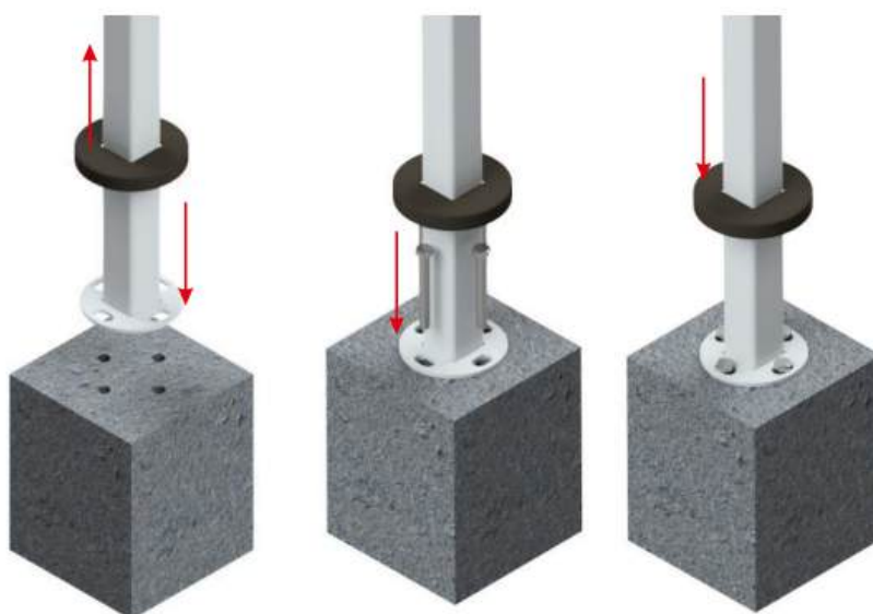
Рисунок 25. Монтаж опоры стрелы
