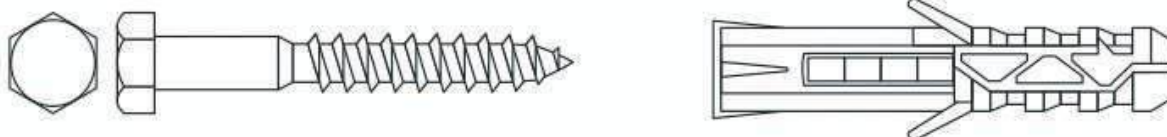
Рисунок 7.4.1 - Шуруп с шестигранной головкой «Глухарь» с дюбелем
