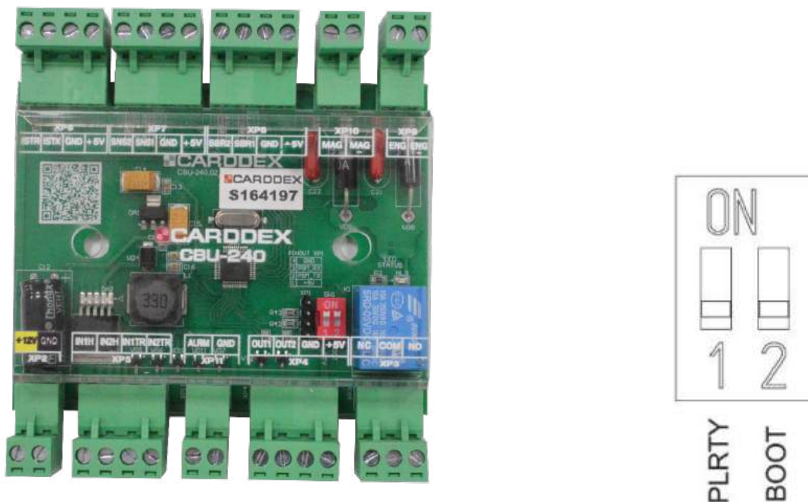
Рисунок 6.3.1 Контроллер управления турникетом «CBU-240» Dip-переключатели
